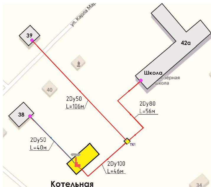
Рисунок 7.4.1. Визуализация отключения участка тепловой сети
