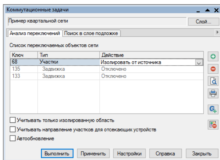
Рисунок 7.2.6. Работа в окне Коммутационные задачи
